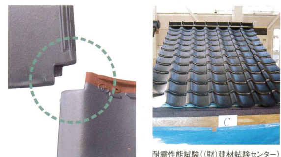
耐震性能試験(財)建材試験センター
