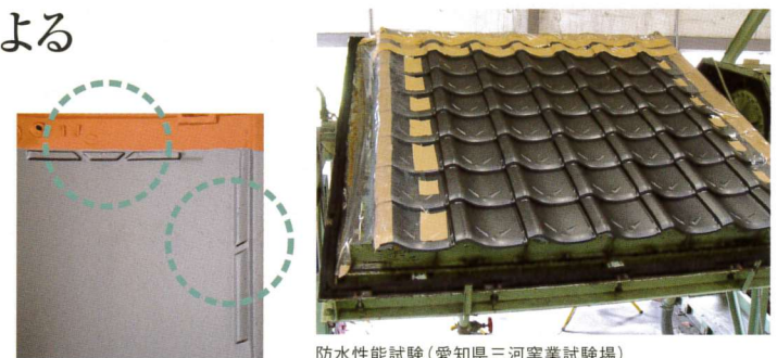
防水性能試験(愛知県三河窯業試験場)
